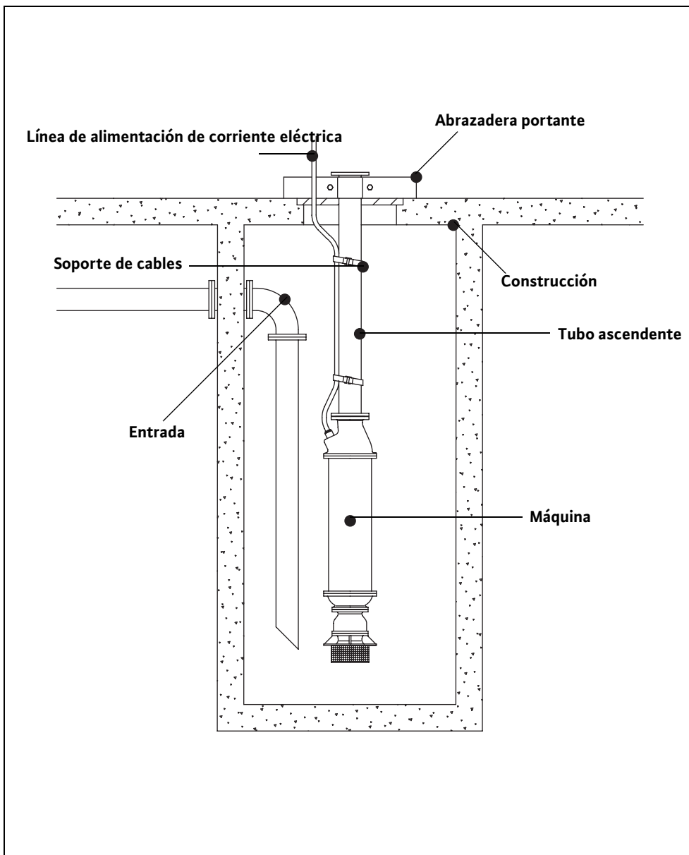
Fig. 5-1: Controlar y rellenar el líquido de llenado del motor
