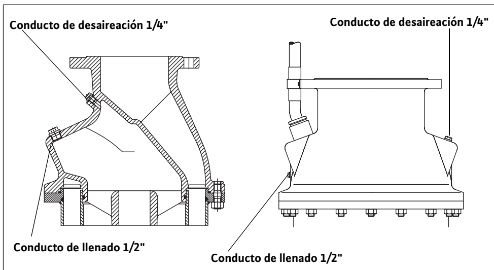
Fig. C-2: Versión antigua y moderna de las conexiones para el conducto de llenado y desaireación
