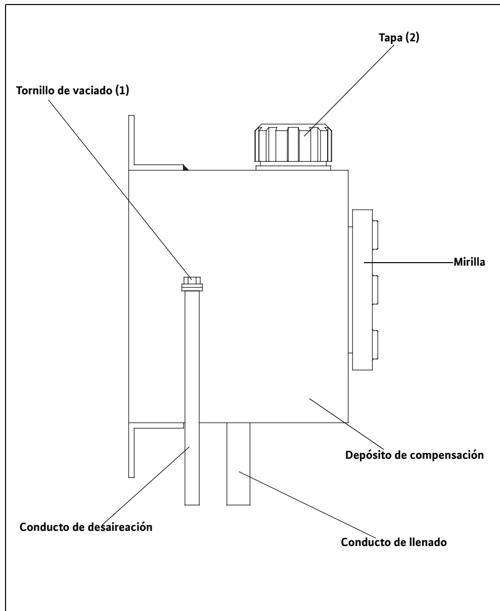
Fig. C-3: Llenado a través del depósito de compensación
